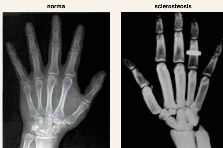
Obr. 1 | RTG – novotvorba kosti (sklerosteóza): defekt v genu SOST nebo v expresi tohoto genu ústí v absenci proteinu sklerostin, což se projevuje mimo jiné zvýšením kostní hmoty.
