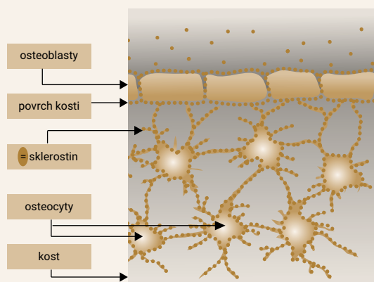
Obr. 2 | Sklerostin ve struktuře kosti: sklerostin secerovaný osteocyty inhibuje blokáci signální dráhy Wnt kostní formaci mediovanou osteoblasty. Upraveno podle [82]
