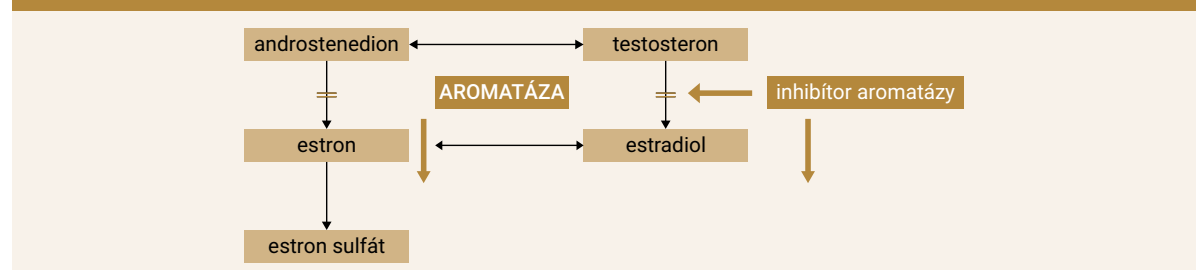
Schéma 2 | Mechanizmus účinku inhibítorov aromatázy
